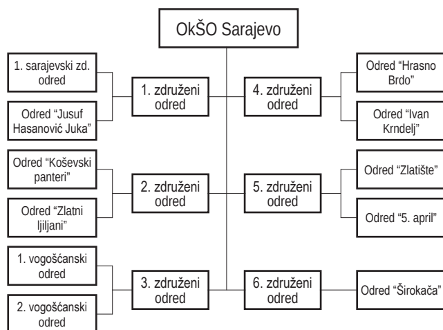
Grafikon 3: OkŠO Sarajevo
